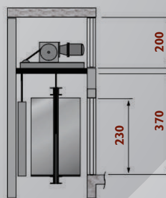
Corte Longitudinal
